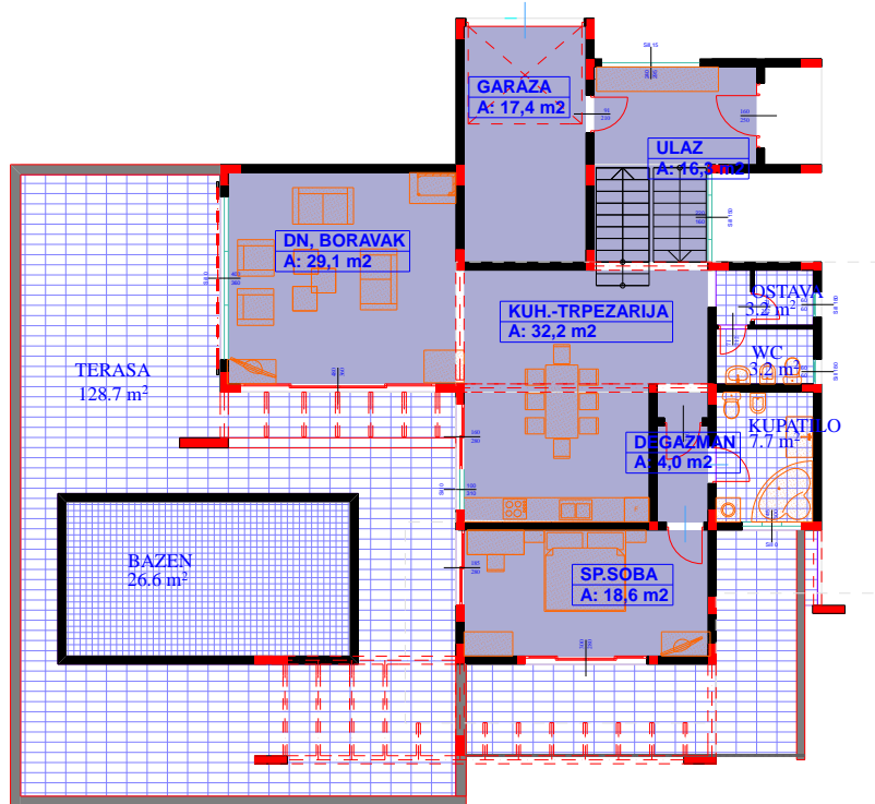
OSNOVA PRIZEMLJA
