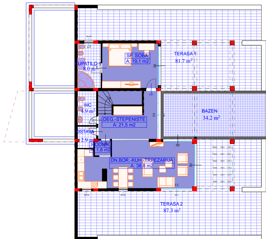
OSNOVA PRIZEMLJA
