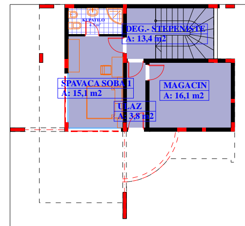
OSNOVA SUTERENA 2
