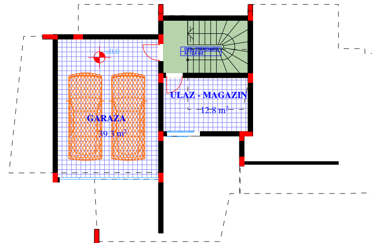
OSNOVA SUTERENA
