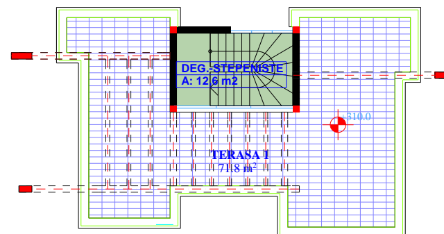
OSNOVA KROVA
