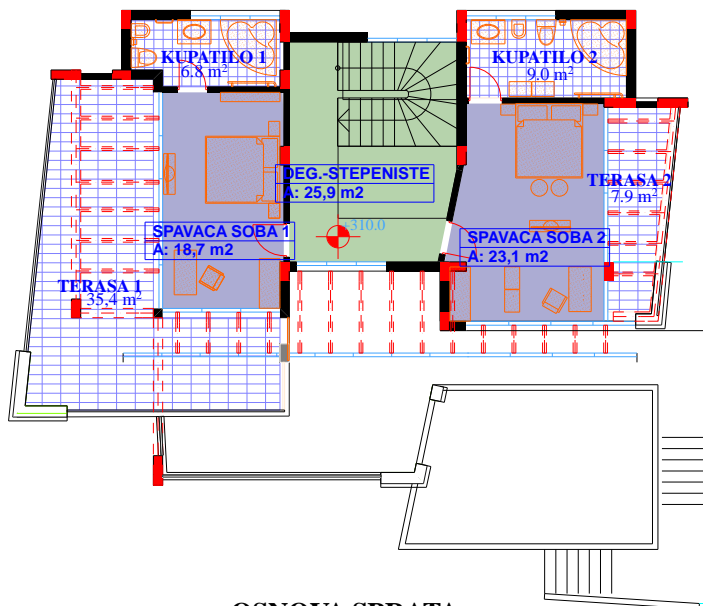
OSNOVA SPRATA
